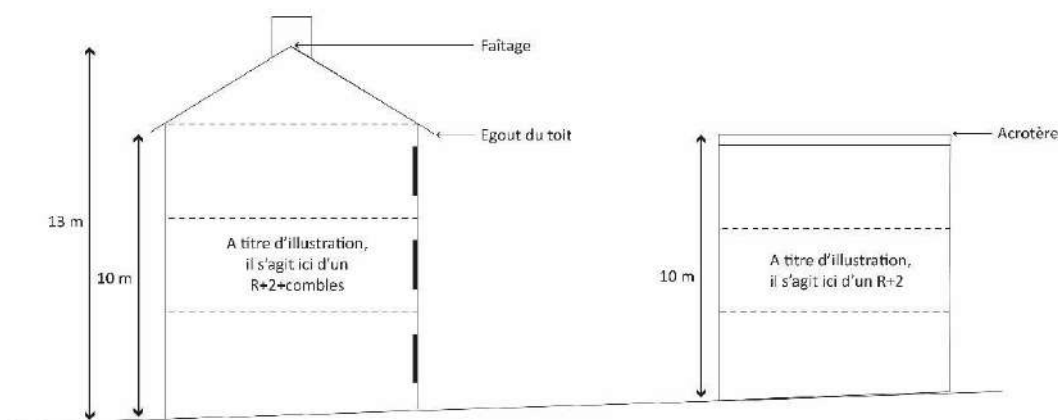
FIGURE 9_Hauteur maximale autorisée en tout point de la construction dans le secteur UB
